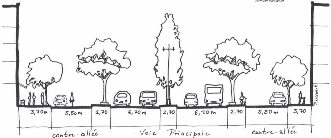
Coupe de l'Octavia Boulevard (situation 2015). © P. Lacroart IAU îdF, d'après Allan Jacobs et Elizabeth Macdonald
